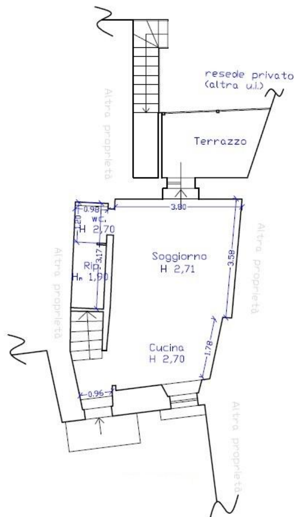
PIANTA PIANO TERRENO
