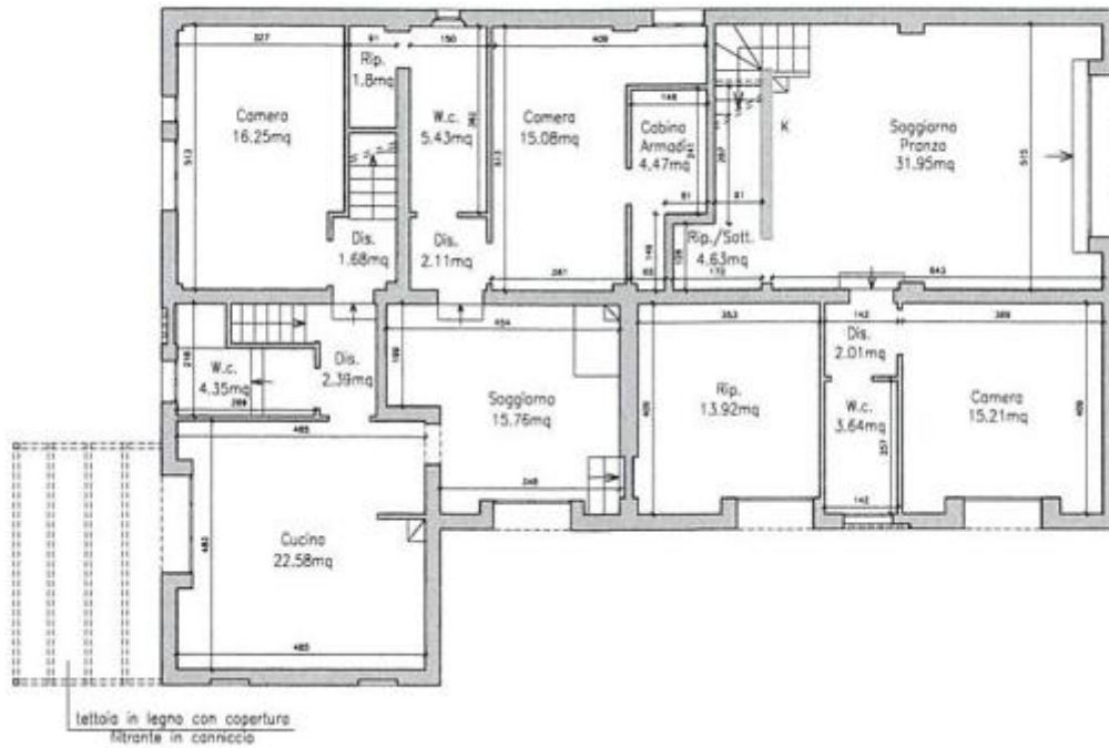
PIANO PRIMO
