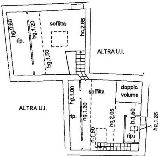
PIANO TERZO
